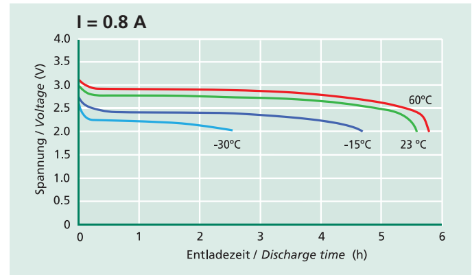
Typische Entladekurven mit Konstantstrom bei verschiedenen Temperaturen Typical discharge curves with constant current at various temperatures
