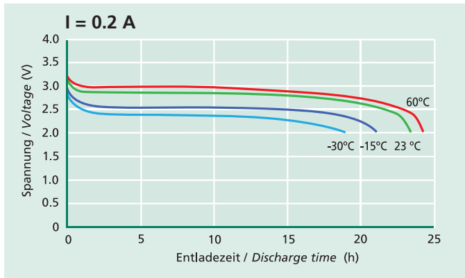
Typische Entladekurven mit Konstantstrom bei verschiedenen Temperaturen Typical discharge curves with constant current at various temperatures
