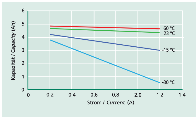
Typische Kapazitätswerte bei verschiedenen Temperaturen Typical capacity values at various temperatures
