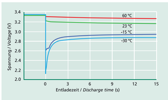
Spannungsverzögerung innerhalb 15 s bei 8 Ohm und verschiedenen Temperaturen Discharge start behaviour 15 s on a 8 Ohm load at various temperatures
